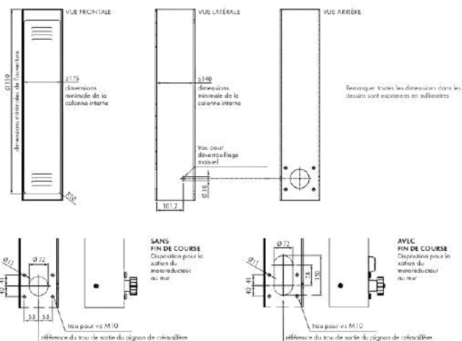
PRÉPARATION POUR L'INSTALLATION DU MOTEUR DANS LA COLONNE
