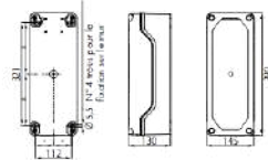
PRÉPARATION POUR L'INSTALLATION DU MOTEUR DANS LA COLONNE
