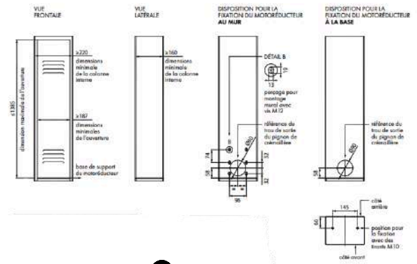
PRÉPARATION POUR L'INSTALLATION DU MOTEUR DANS LA COLONNE
