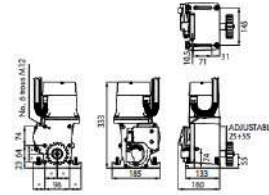
DIMENSIONS MOTEUR
