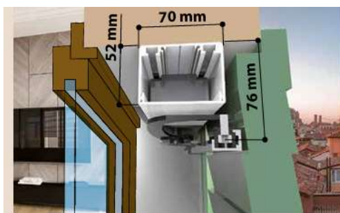
Dimensions coupe RHA
