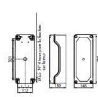
DIMENSIONS CENTRALE DE COMMANDE
