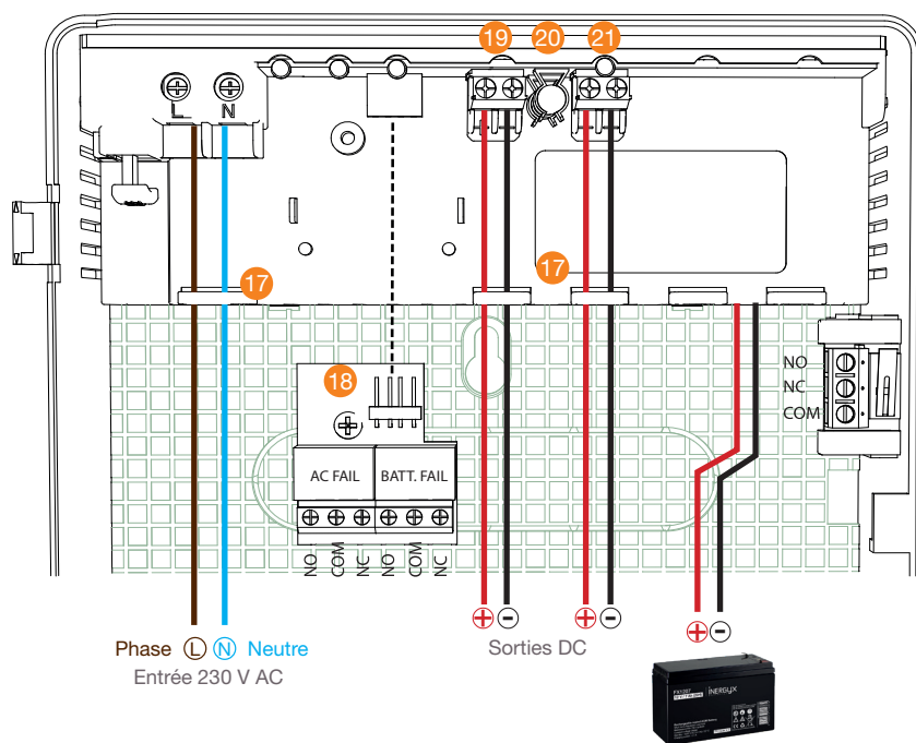
Batterie INERGYX 12V 7Ah réf. FX1207 ou équivalente
