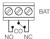
Relais représenté en mode défaut batterie ou tension seuil bas (10.5-11V DC) ou absence batterie.
