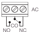
Relais représenté en mode absence secteur
